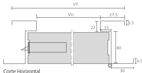
Corte Horizontal Horizontal cut Coupe horizontal
